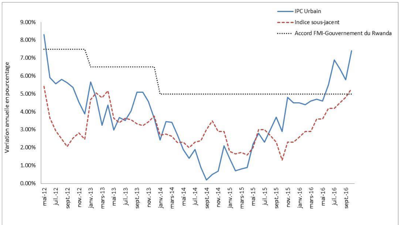
Graphique 1: Variation annuelle de l'IPC (Mai 2012– Octobre 2016)
